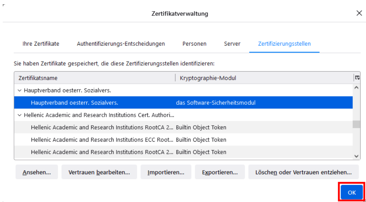
Abbildung 9: Zertifikatverwaltung – Kontrolle
