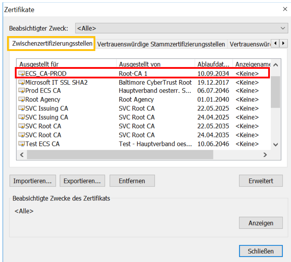
Abbildung 11: Zertifikatsübersicht "Zwischenzertifizierungsstellen"
