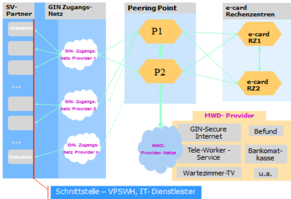
Abbildung 2: Struktur des GIN
