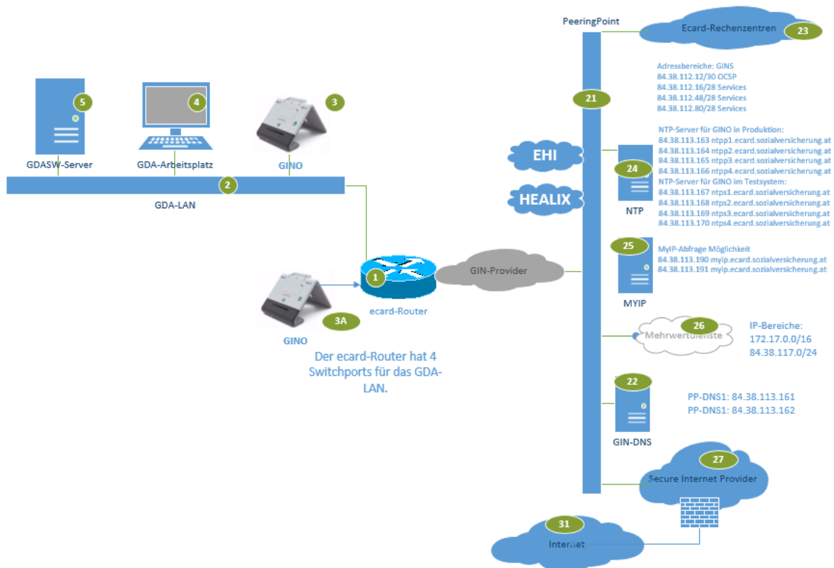
Abbildung 19: Minimalsetup eines VP-LANs mit e-card-Anschluss
