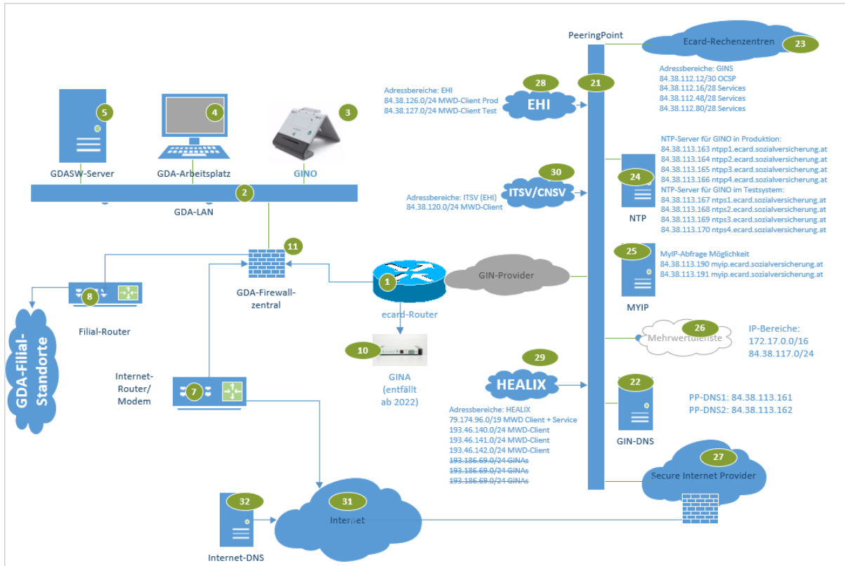
Abbildung 24: „Gesamtübersicht eines Vollausbauens“ mit Filialen und lokalem Internet-Anschluss
